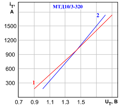
Рисунок 1: Предельные вольтамперные характеристики при максимально допустимой температуре перехода T_{jm} (1) и температуре T_j=25\text{ }^\circ\text{C} (2), I_T=3,14 I_{TAV} .
