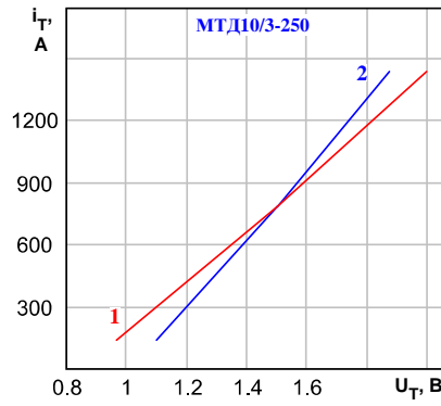
Рисунок 1: Предельные вольтамперные характеристики при максимально допустимой температуре перехода T_{jm} (1) и температуре T_j=25\text{ }^\circ\text{C} (2), I_T=3,14 I_{TAV} .
