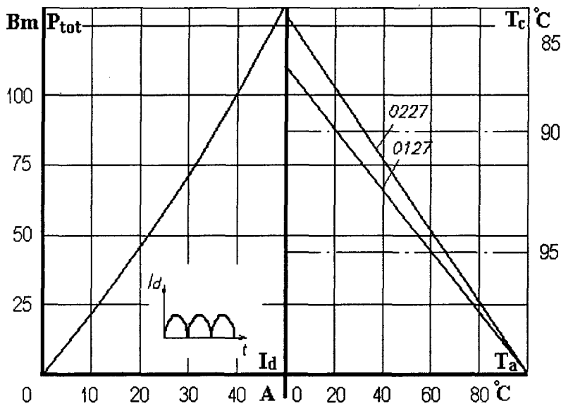
* Рис. 2. 52. Зависимость допустимой суммарной рассеиваемой мощности и допустимого выпрямленного тока двух модулей МТОТО4/3 - 63 на охладителях О127 и О227 от температуры окружающей среды и температуры корпуса при естественном охлаждении
