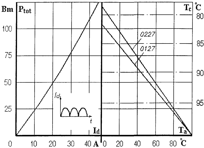
* Рис. 2. 49. Зависимость допустимой суммарной рассеиваемой мощности и допустимого выпрямленного тока двух модулей МТОТО4/3 - 40 на охладителях О127 и О227 от температуры окружающей среды и температуры корпуса при естественном охлаждении
